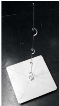
Figura 4.13: La antena omni colineal completa
